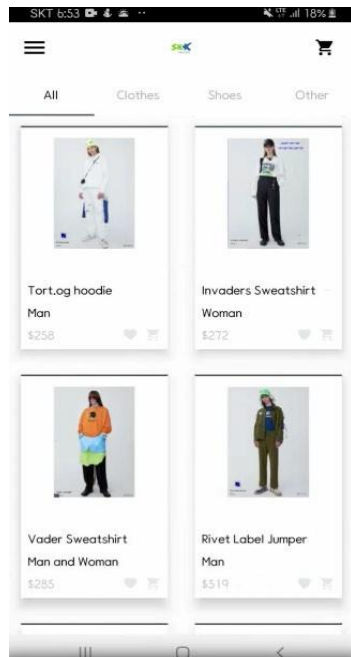
item list
